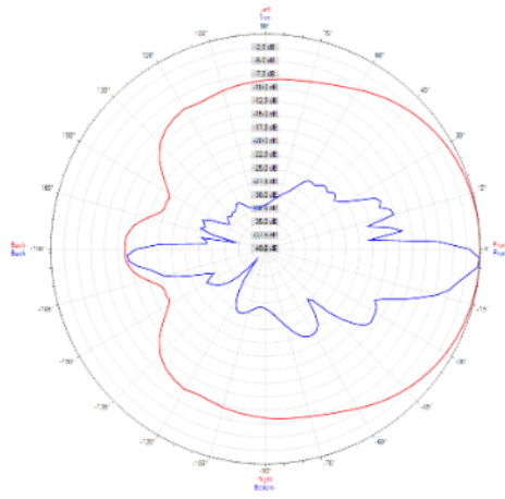
2 kHz 1/3 Oct
