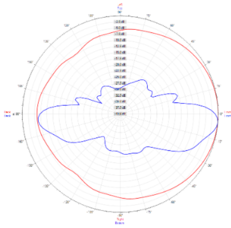
1 kHz 1/3 Oct
